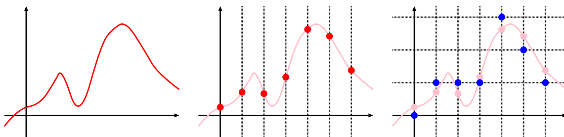
横軸が変数, 縦軸が値. 左から, 元のデータ (曲線), それを標本化したもの (赤点), さらに量子化したもの (青点)
