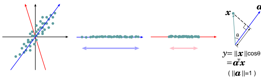
図 3: 左端の図に灰色で示された 2 次元データを青い軸方向の成分のみで説明しようとする、その成分は左から 2 番目の図のように散らばる。赤い軸方向の成分のみだと、左から 3 番目の図のように散らばる。
