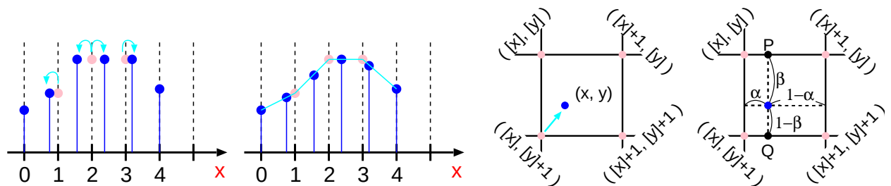
図 2: 最近傍法と線形補間法。左の 2 つは最近傍法／線形補間法による 1 次元パターンの補間を示し、右の 2 つは最近傍法／線形補間法による画素値の補間の例を示す。
